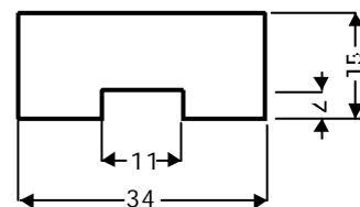
U11 ①
