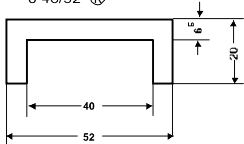
U 40/52 ®
