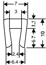
Perfil "U3" ®
