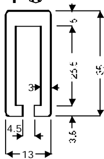
UCLIP I ®
