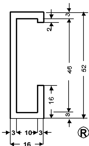
Denominación: C 46
