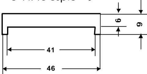
U 41/46 esp.6 ®
