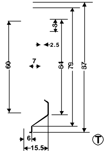
BarandaH87
