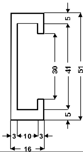
Denominación: C 46
