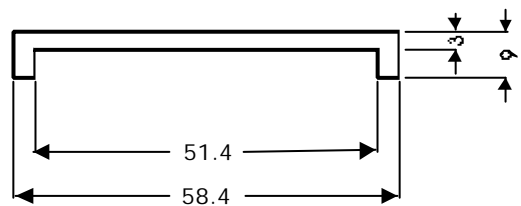
U50 ®
