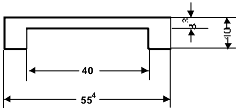
U 40/55 ®
