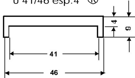
U 41/46 esp.4 ®
