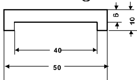
U 40 ®
