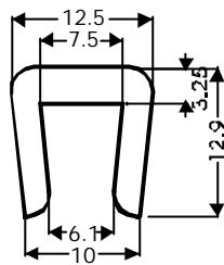
PERFILU1/4" ®
