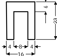
U 8 ①
